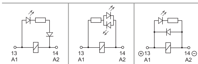
C: Опция 3, 5, 54 светодиод (AC)
